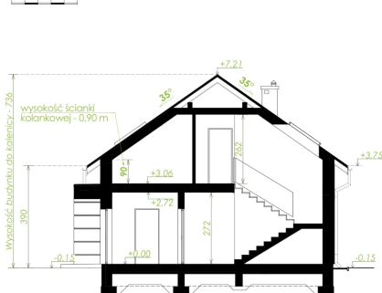
PRZEKRÓJ SKALA 1:100 PA - 10
