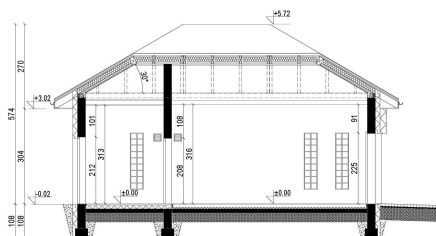
HomeKONCEPT-G 04 wersja podstawowa Przekrój BB
